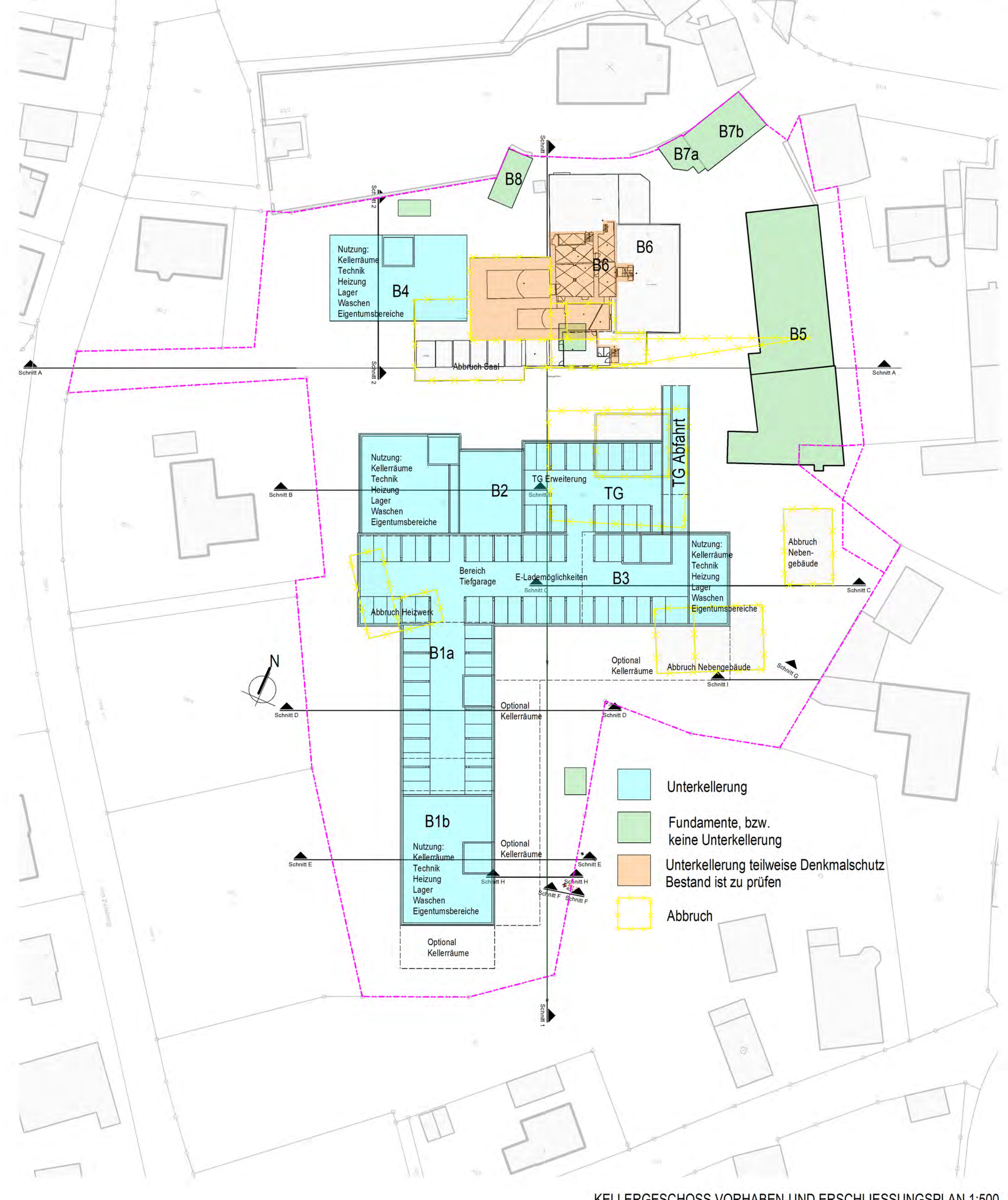
KELLERGESCHOSS VORHABEN-UND ERSCHLIESSUNGSPLAN 1:500
